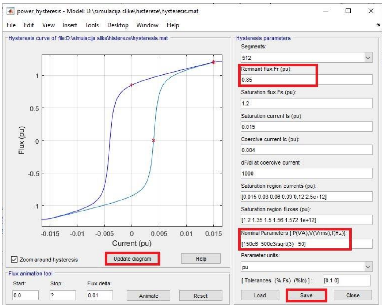
Slika 6.7. Oblikovanje petlje histereze.
