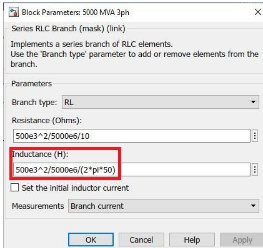
Slika 6.3. Prozor RL serijske grane.
