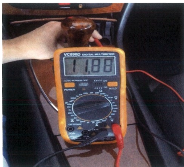
Slika 2.1.2 Mjerenje napona potrošača (upaljač) u automobilu
