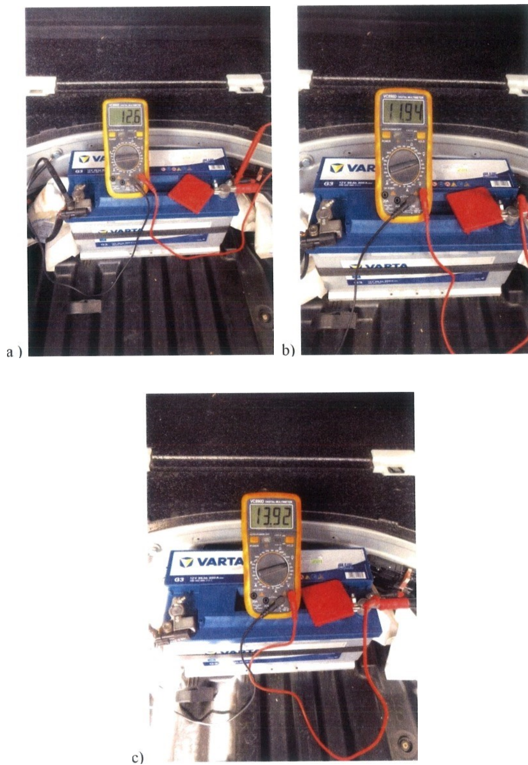
Slika 2.2.3 . Napon akumulatora u ,stanju mirovanja ( slika a), napon akumulatora pri pokretanju (slika b), napon akumulatora nakon uсталjenog stanja (slika c)
