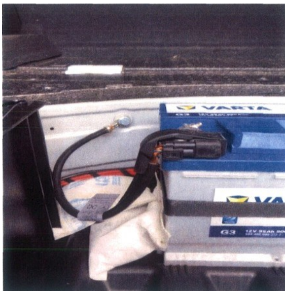
oblika 2.2.2. Spoj negativne priključnice automobil. Ake baterije s korosć•rijom
