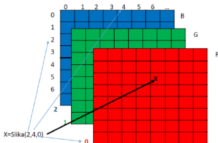
Sl. 2.4. Zapis RGB slike pomoću polja s tri dimenzije.
