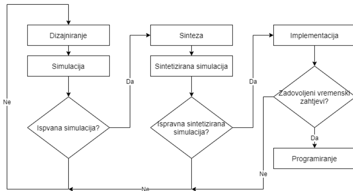
Sl. 3.11. Dijagram toka izrade FPGA sustava.
