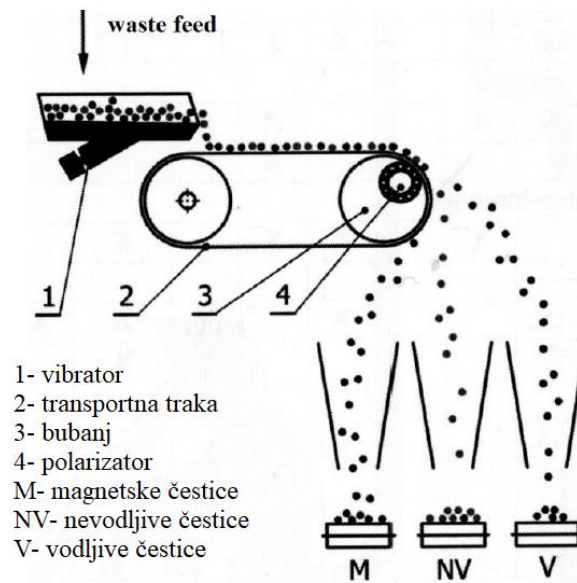
Slika 2.12. Razvrstavanje vrtložnim strujama [7]
