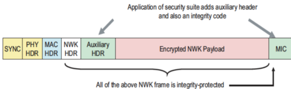
Slika 3.7 ZigBee okvir sa zaštitom na mrežnom sloju [8]
