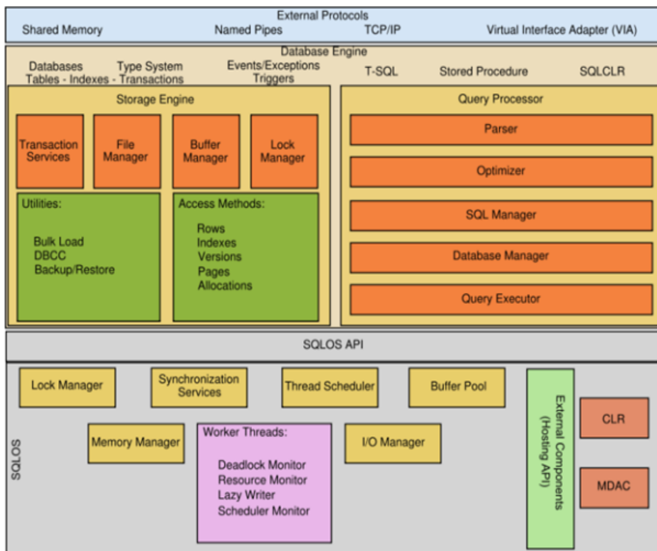
Slika 3.3. Arhitektura Microsoft SQL Servera [11]
