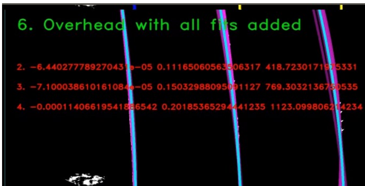
Slika. 3.13. Prikaz detektiranih linija na binarnoj slici s pripadnim koeficijentima krivulja polinoma koje označavaju linije vozne trake.
