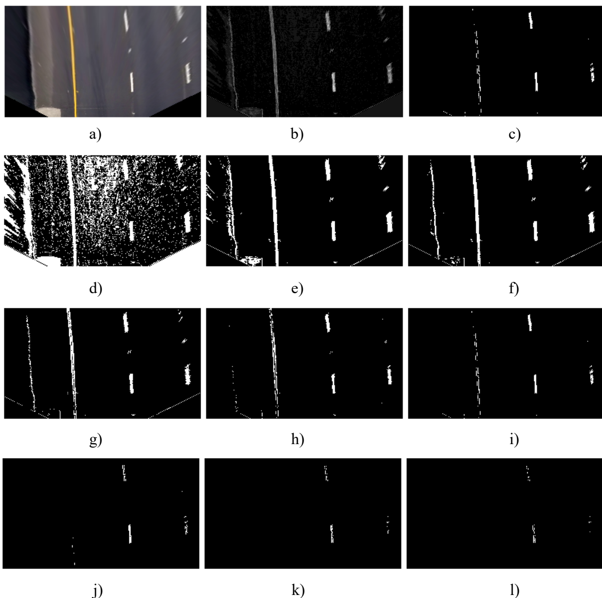
Slika. 3.8. Dobivanje binarne slike primjenom 22 razliĉita filtra (a) slika podruĉja interesa (ROI) iz ptiĉje perspektive koja se obraĊuje filtrima; (b) konaĉna binarna slika dobivena kombinacijom svih 22 filtra; (c) konaĉna binarna slika dodatno filtrirana kroz automatsku izraĉunatu vrijednost gornje granice filtriranja 6; (d)-(l) konaĉna binarna slika dodatno filtrirana uz vrijednosti gornje granice filtriranja: 1,2,3,4,5,6,7,8 i 9.
