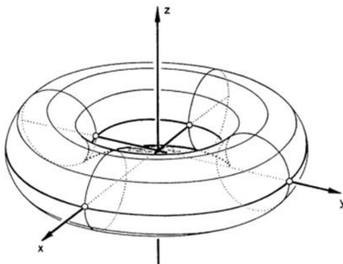
Slika 2.4. Torus of revolution [3]
