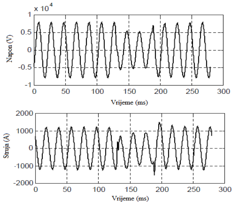
Slika 6.7. Poremećaj uslijed propada napona[8]
