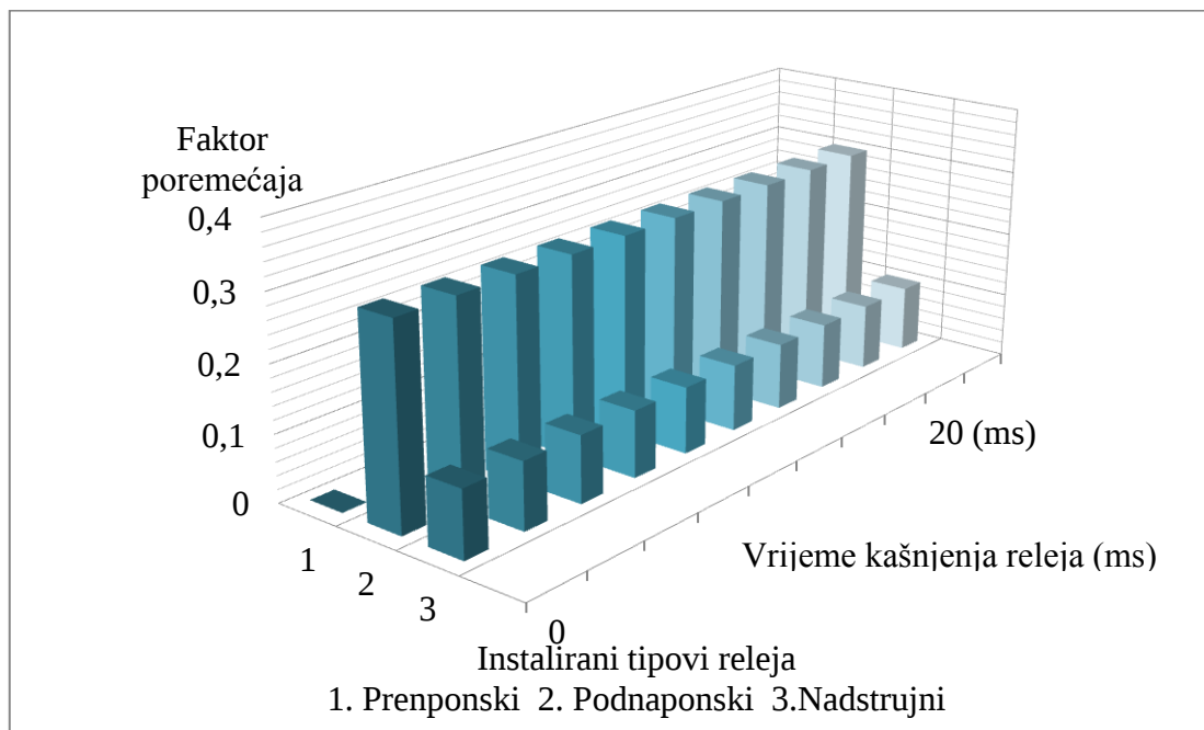
Slika 6.8. Utjecaj propada napona na zonu podešavanja releja
