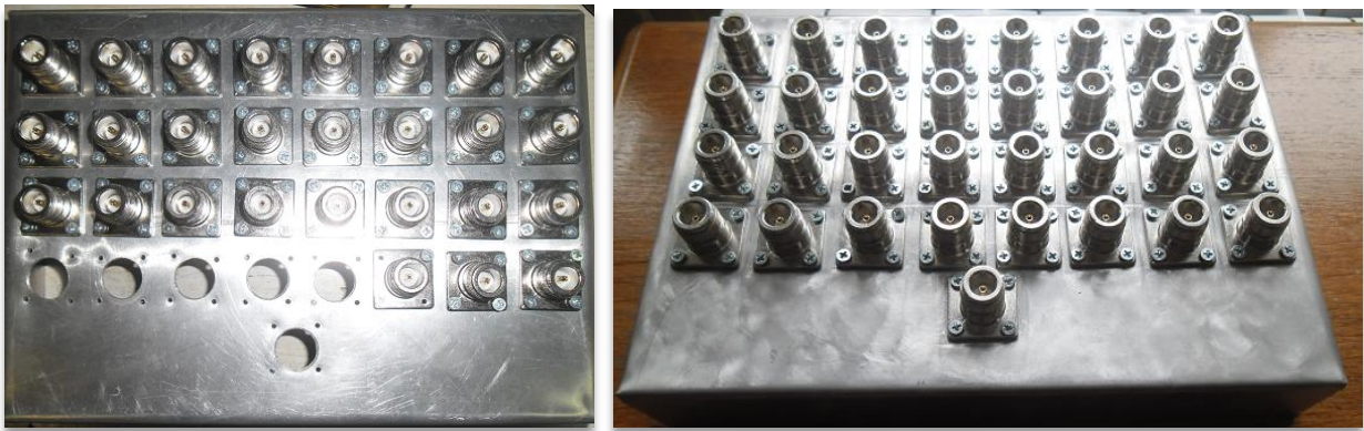
Slika 3.11. Izgled kućišta s djelomično postavljenim konektorima, konačan izgled kućišta.
