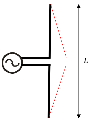
Slika 3.6. Kratki dipol
