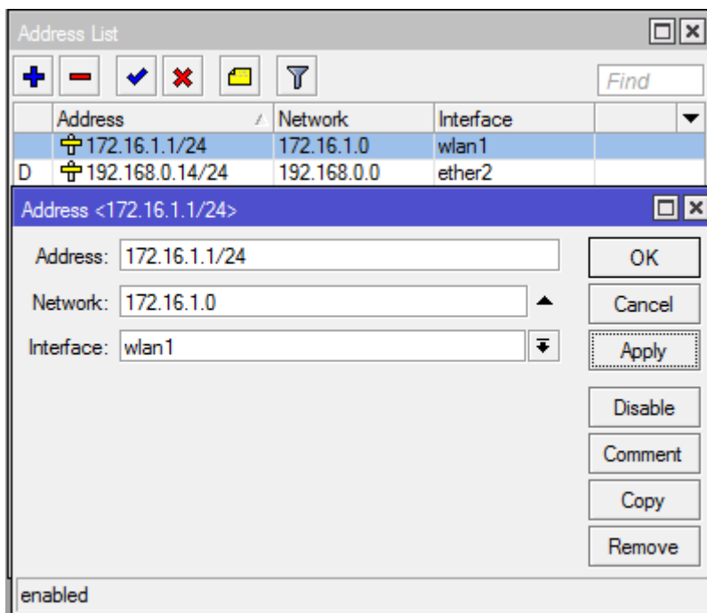
Slika 4.7. Prikaz opcije Address u Winbox-u
