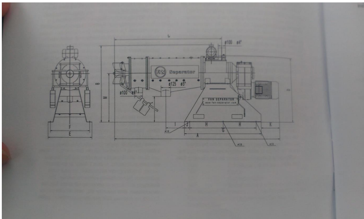
Slika 5.11. Shema separatora
