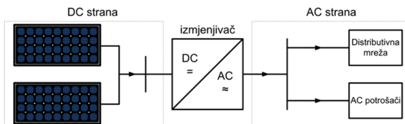
Slika 2.15. FN sustav spojen na mrežu [2]
