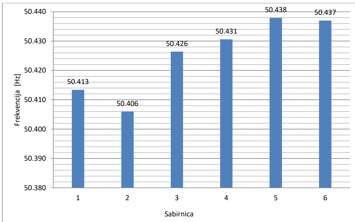
Slika 4.8. Najveće odstupanje frekvencije od nominalne za 1. slučaj VE snage 60 MW na različitim sabirnicama u mreži
