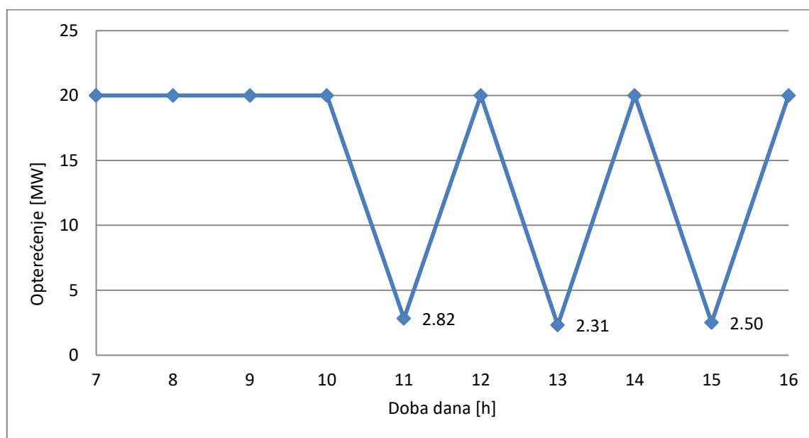
Slika 4.11. Opterećenje na mrežu dijela potrošača s ugrađenim podfrekvencijskim relejima
