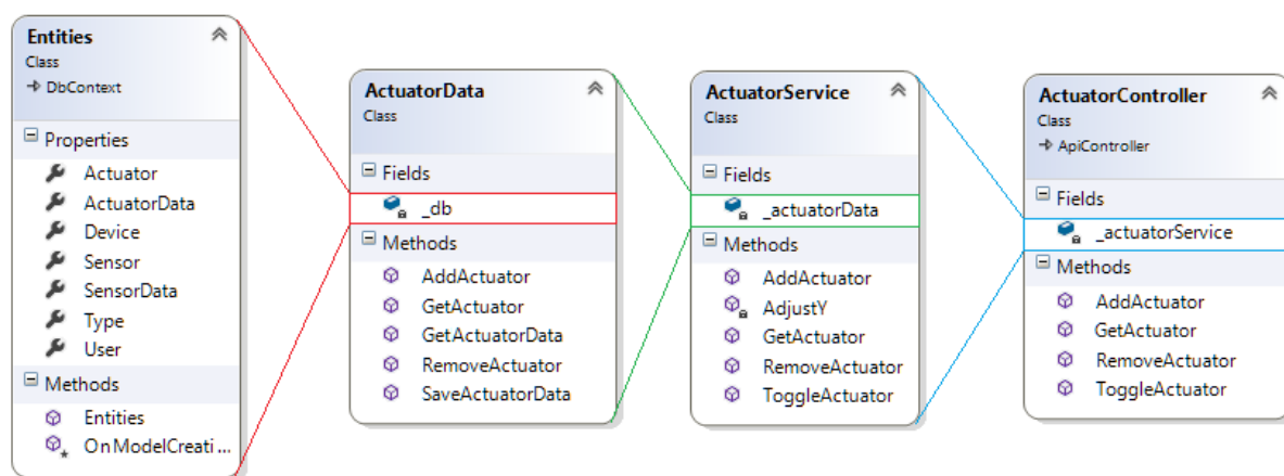
Sl. 4.5. Dijagram klasa.
