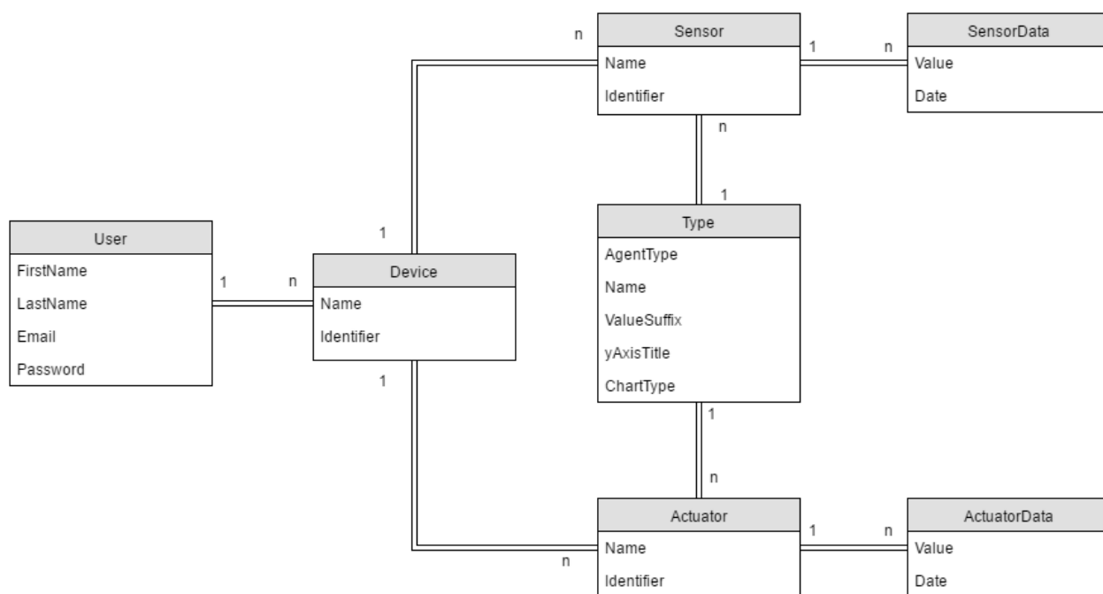
Sl. 4.2. ER dijagram konceptualnog modela.
