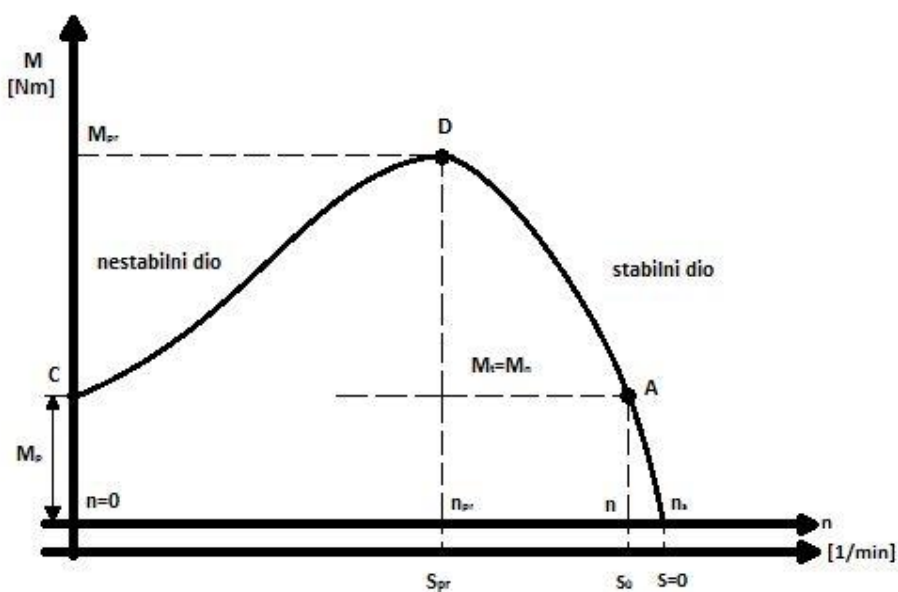
Slika 4.10. Momentna karakteristika asinkronog motora
