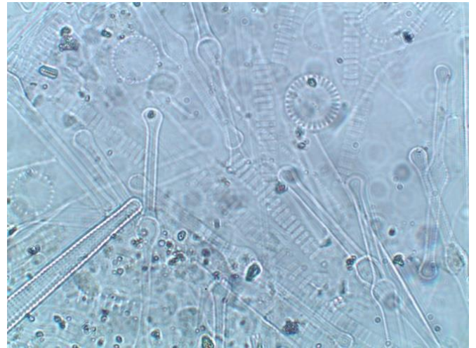
Slika 9.2. Stephanodiscus hantzschii (desno) i Cyclotella meneghiniana (lijevo)
